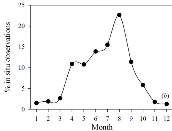
Número de observaciones in situ al año (sup.) y distribución de muestras por mes (inf.).
