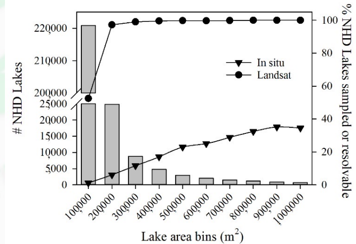
Porcentaje de lagos muestreados por área superficial
