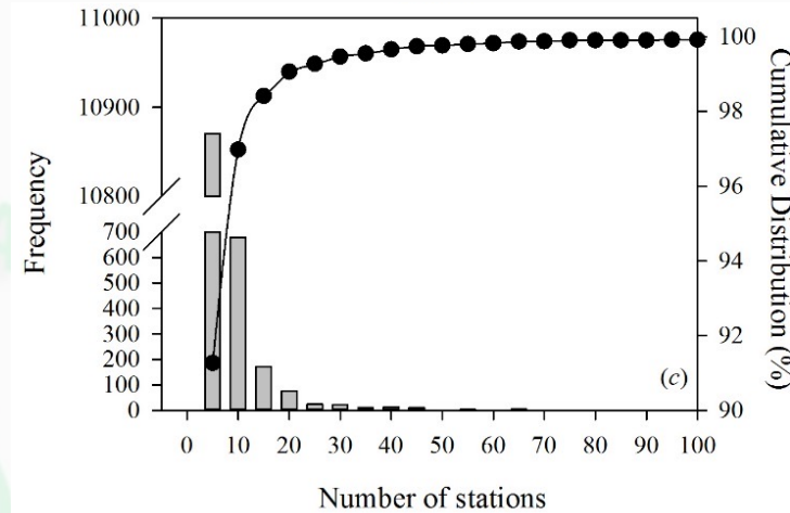
Número de estaciones por lago y distribución acumulativa por lago.
