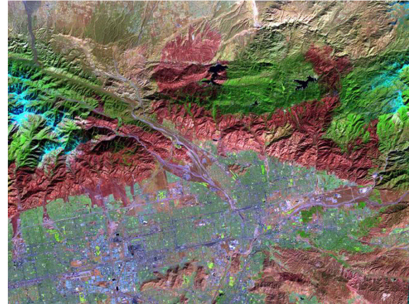
Imagen ASTER del incendio Old Fire / Grand Prix 2003 al este de Los Ángeles. Credito de imagen: NASA
