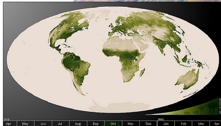
Satélite Suomi NPP (arriba); Mapa global de vegetación (izquierda). Credito de imagen: NASA/NOAA
