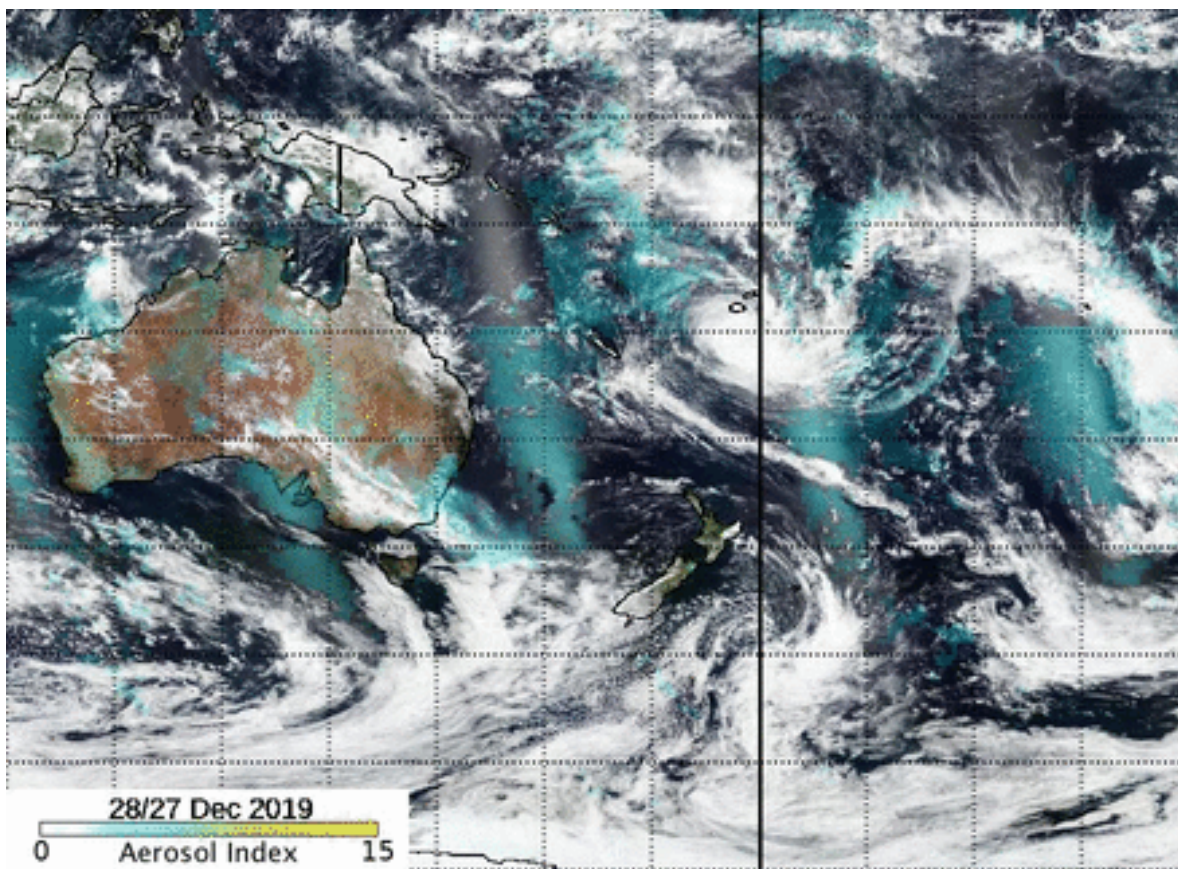
Los instrumentos VIIRS y OMPS-NM rastrean el movimiento del humo de los recientes incendios australianos (izquierda); VIIRS detecta ubicaciones activas de incendios a lo largo del este de Australia (derecha). Credito de imagen: NASA
