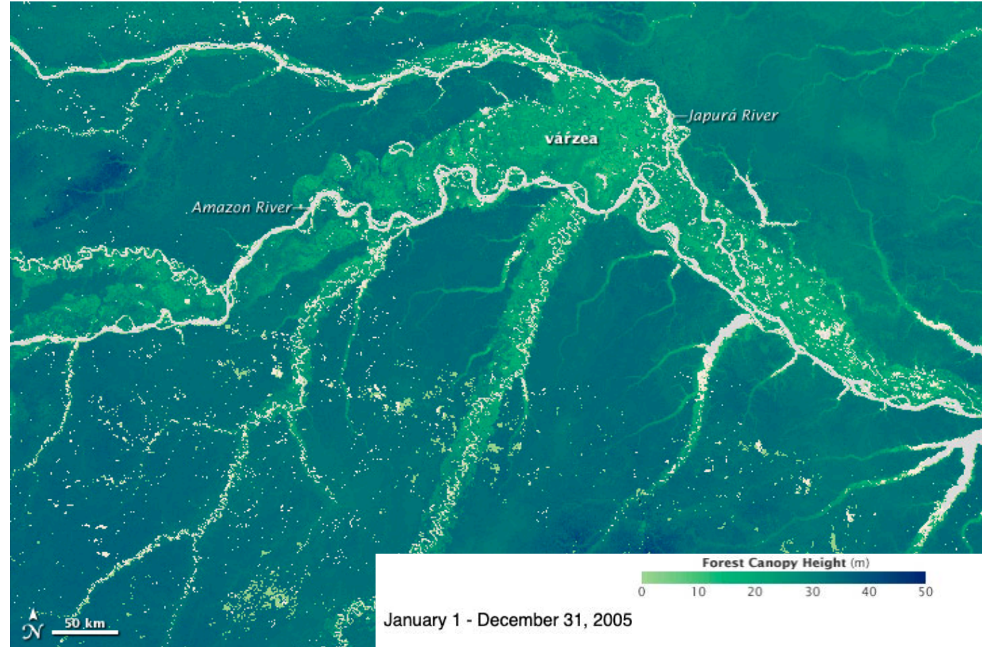
Altura del dosel del bosque (sensores múltiples). Credito de imagen: NASA
