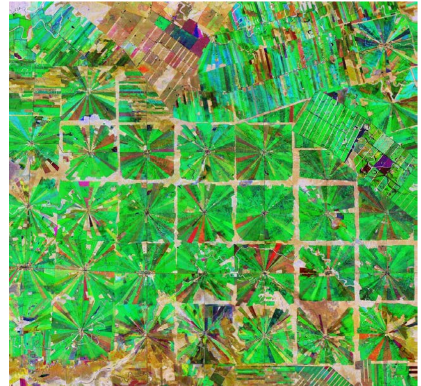
Imagen compuesta de Sentinel-2 de bosques convertidos en tierras de cultivo en Brasil 2019. Crédito de la imagen: ESA
